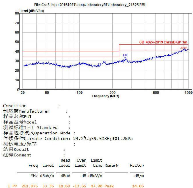
图 4-5 RE 测试水平方向
