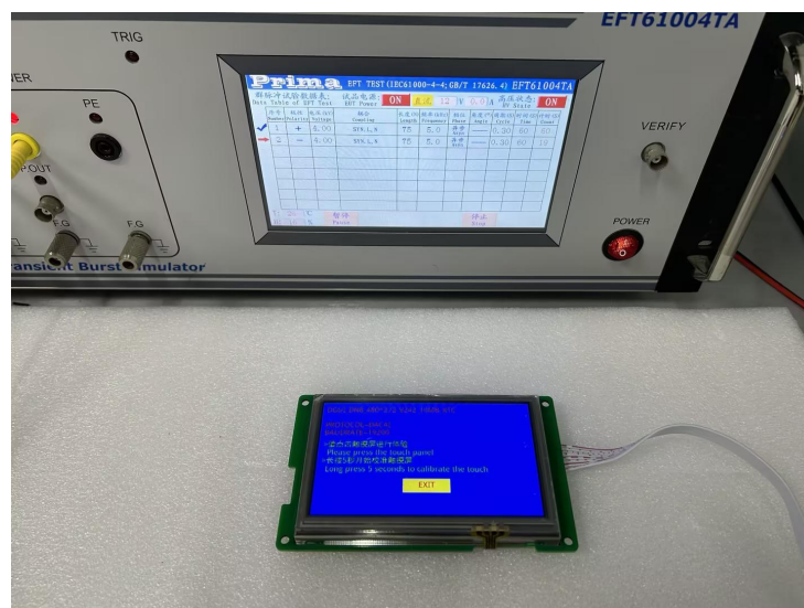
图 4-3 EFT 测试图
