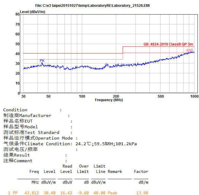
图 4-6 RE 测试垂直方向
