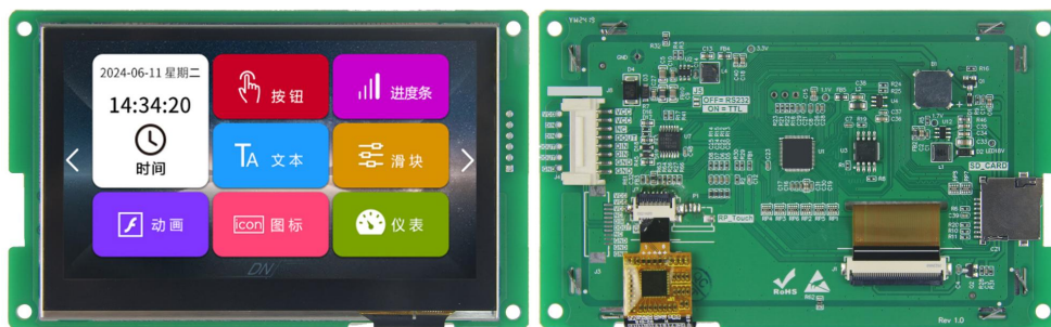
图 1-2 4.3 寸电容触摸参考图
