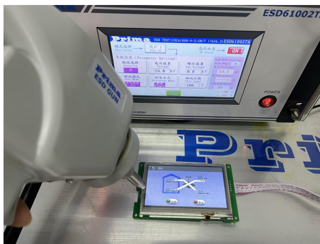
图 4-2 ESD 测试图
